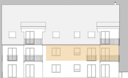
Ansicht Westen
