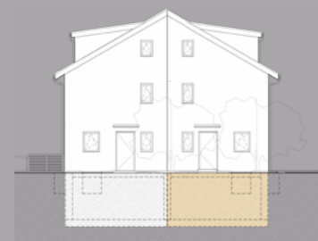
Ansicht Nord
