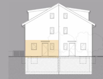
Ansicht Nord
