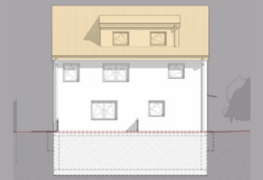
Ansicht Ost
