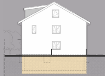
Ansicht West
