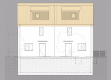
Ansicht Nord
