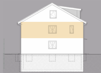
Ansicht Ost
