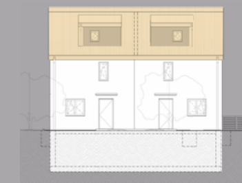
Ansicht Nord
