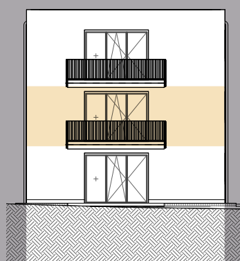
Ansicht West
