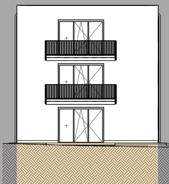
Ansicht West
